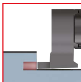
7 AUSSENPLANEIN- STECHEN
