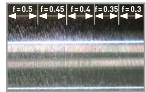
Herkömmlich
